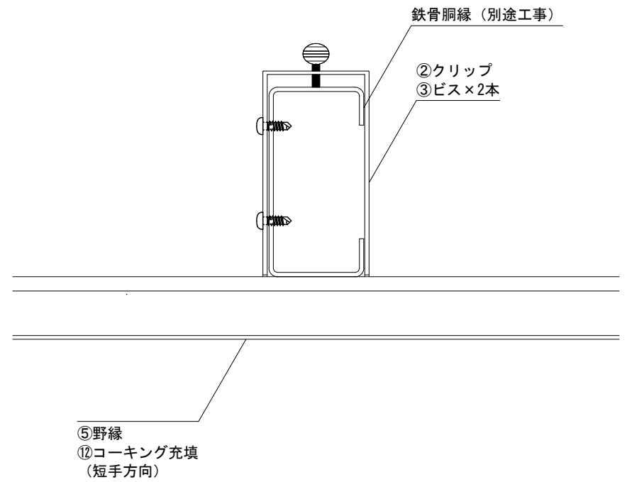
【鉄骨胴縁並行方向】
